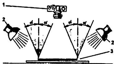
Схема расположения источников света при репродукционной фотосъемке. Цифрами обозначены: 1 — фотокамера; 2 — осветители; 3 — оригинал. Обозначение 2d показывает угол поля зрения объектива.
