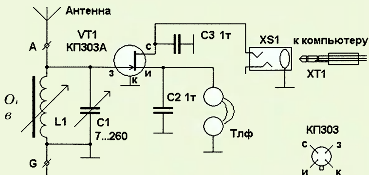
Схема приемника на одном транзисторе.
